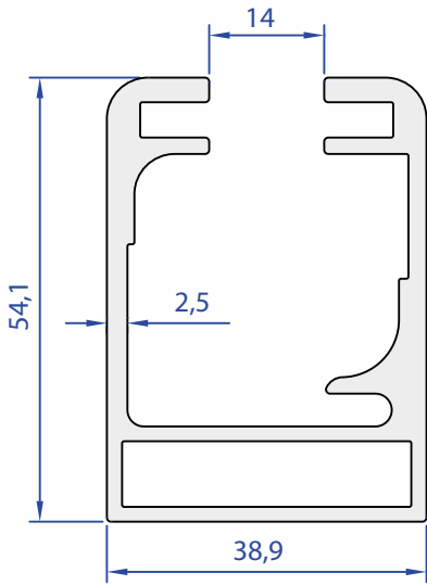
75116-00 1,445 Kg/m
