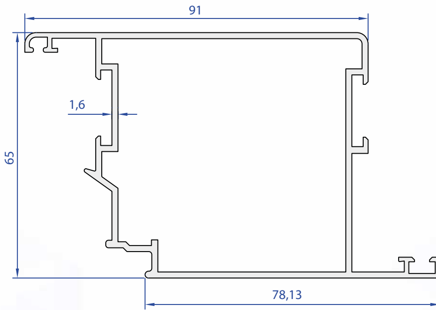
81011-00 1,509 Kg/m
