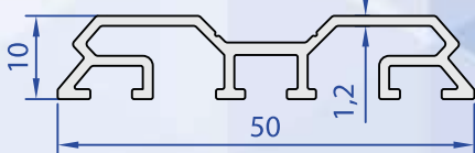
83010-00 0,372 kg/m
