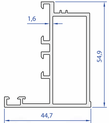
81016-00 0,879 Kg/m
