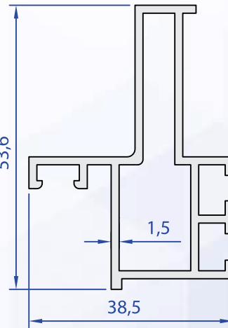
83002-15 0,775 kg/m
