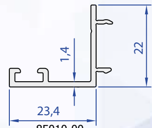
85010-00 0,226 Kg/m
