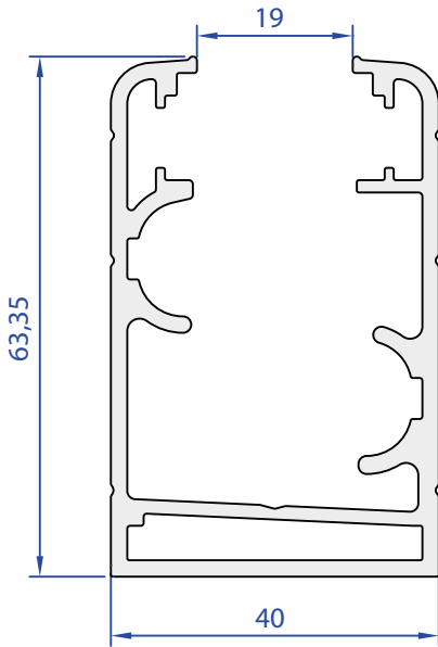
75472-00 1,439 Kg/m
