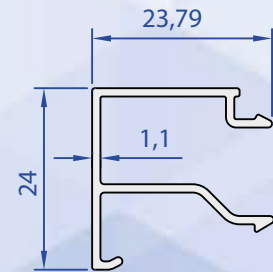
85003-00 0,238 Kg/m
