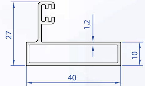
75324-00 0,435 Kg/m
