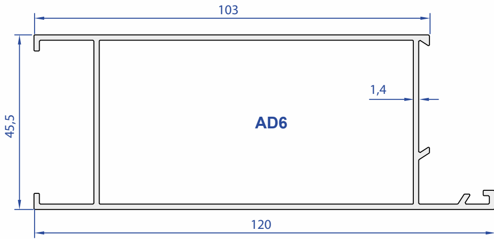
AD6 80011-14 1,240 kg/m
