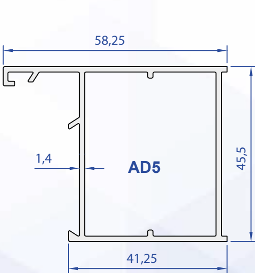
AD5 80012-14 0,759 Kg/m
