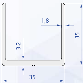
85006-00 0,607 Kg/m
