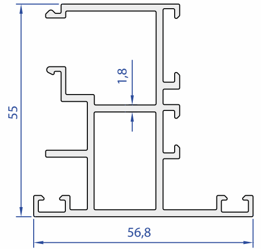
81014-00 1,168 Kg/m
