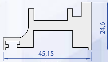
05055-00 1,126 kg/m
