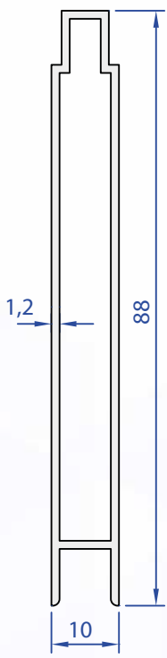
80001-12 0,621 kg/m
