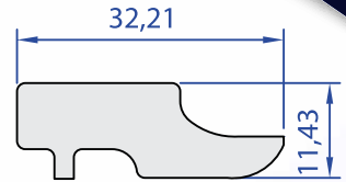
83004-00 0,669 kg/m
