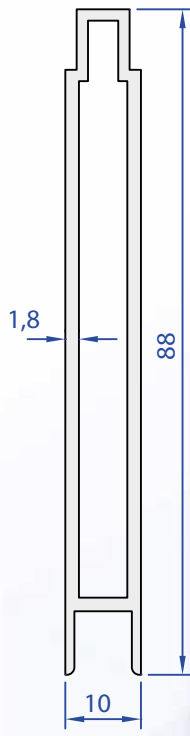
80001-18 0,874 kg/m
