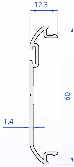
85009-00 0,333 Kg/m
