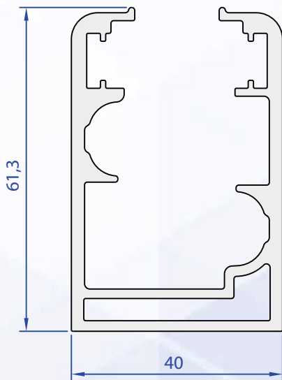
75397-00 1,532 Kg/m
