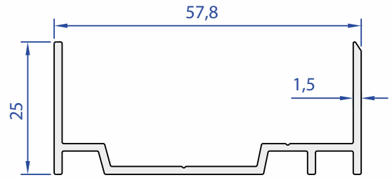
40130-00 0,462 Kg/m
