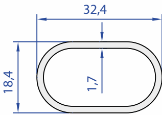
40191-00 0,370 Kg/m
