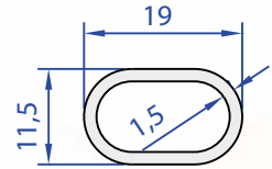
40194-00 0,189 Kg/m
