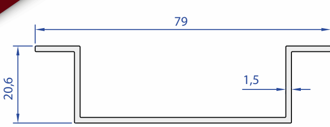
40131-00 0,477 Kg/m
