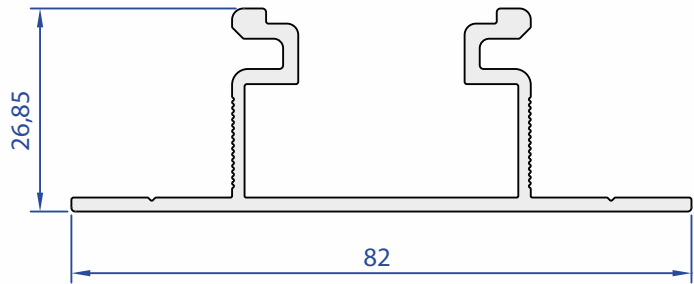
40209-00 0,803 Kg/m
