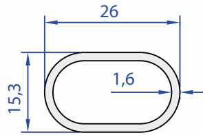
40192-00 0,279 Kg/m
