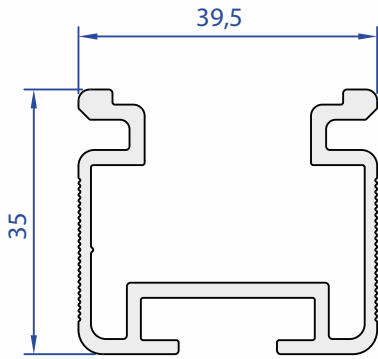
40210-00 0,792 Kg/m
