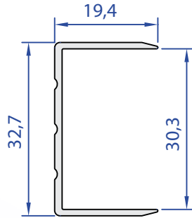
60413-00 0,228 Kg/m
