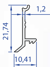
60052-00 0,099 kg/m
