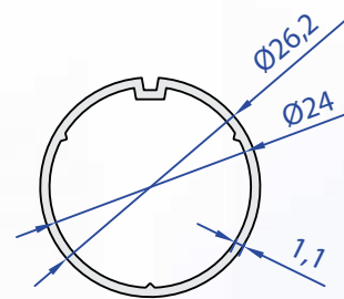
60094-00 0,244 kg/m
