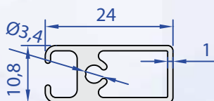
60087-00 0,253 kg/m
