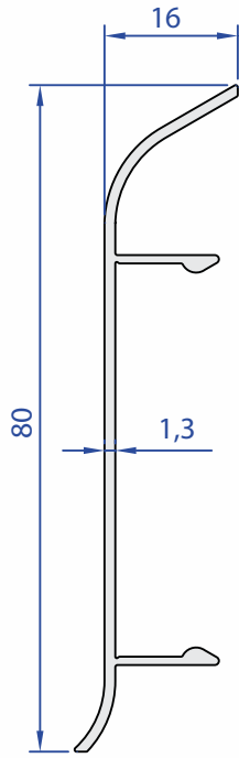
05715-00 0,391 Kg/m
