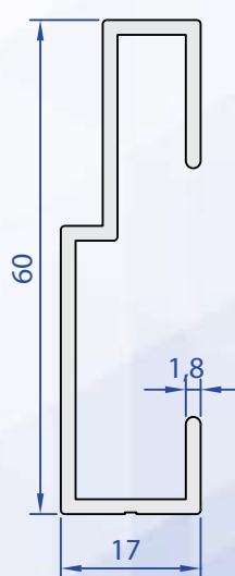
60112-00 0,565 kg/m
