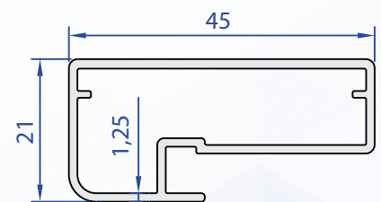
60225-00 0,476 Kg/m
