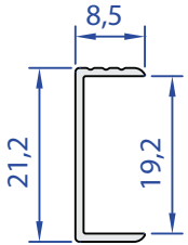
60429-00 0,095 Kg/m
