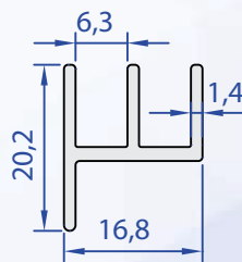
60135-00 0,222 kg/m
