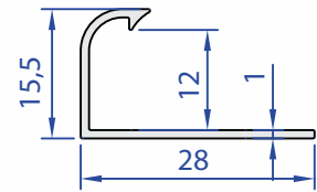
60072-00 0,132 kg/m
