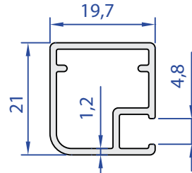
60277-00 0,282 Kg/m
