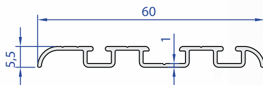
60390-00 0,270 Kg/m
