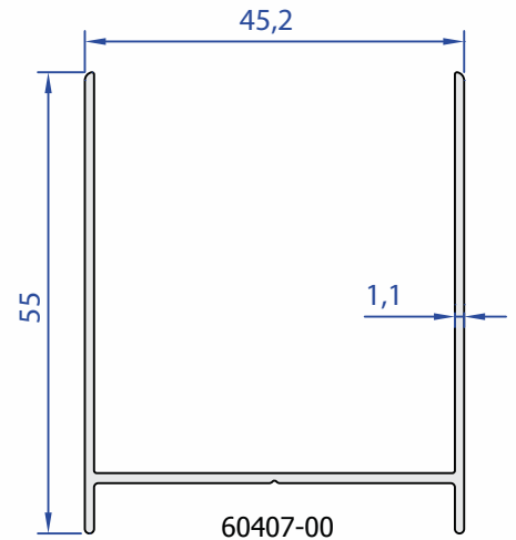
60407-00 0,466 Kg/m
