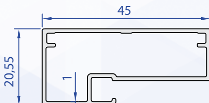
60433-00 0,390 Kg/m
