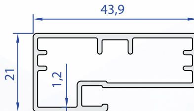
60274-00 0,506 Kg/m
