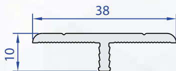
60555-00 0,294 Kg/m
