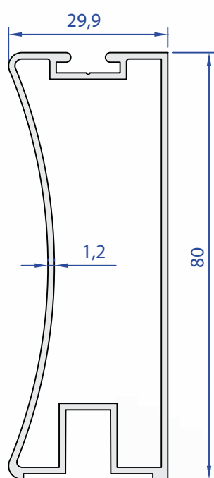
60006-00 0,827 kg/m
