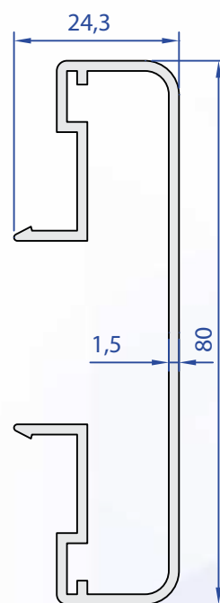
60009-00 0,761 kg/m
