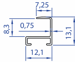
60185-00 0,074 kg/m
