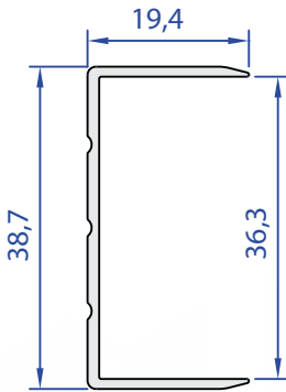
60466-00 0,251 Kg/m
