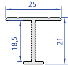
60363-00 0,191 Kg/m
