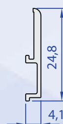
60044-00 0,118 kg/m
