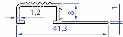
60084-00 0,210 kg/m
