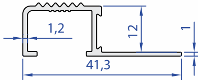
60086-00 0,236 kg/m
