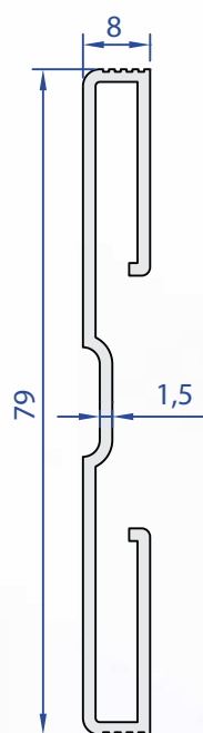
60007-00 0,567 kg/m
