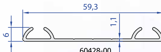
60428-00 0,254 Kg/m
