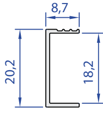
60173-00 0,091 kg/m
