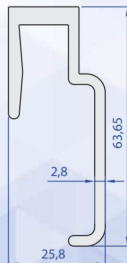
60113-00 0,992 kg/m
