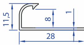
60032-00 0,121 kg/m
