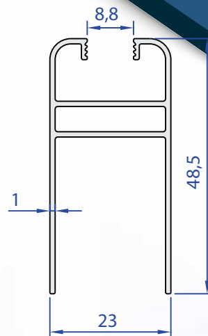
60441-00 0,417 Kg/m
