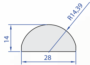
60129-00 0,847 kg/m
