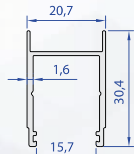
60111-00 0,283 kg/m
