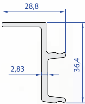
60572-00 0,438 Kg/m
