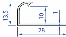
60031-00 0,127 kg/m
