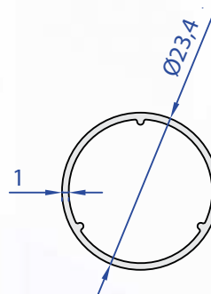
60459-00 0,280 Kg/m
