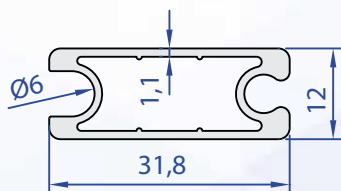
60107-00 0,334 kg/m
