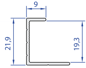
60454-00 0,168 Kg/m
