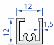
60011-00 0,174 kg/m
