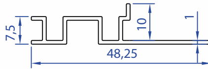
60036-00 0,224 kg/m
