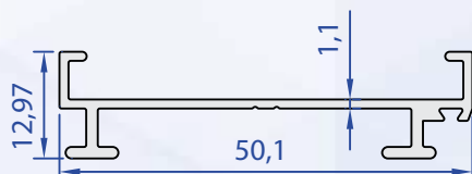
60104-00 0,292 kg/m
