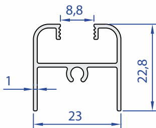
60443-00 0,247 Kg/m
