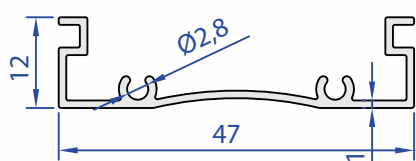
60128-00 0,260 kg/m
