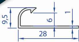
60071-00 0,116 kg/m
