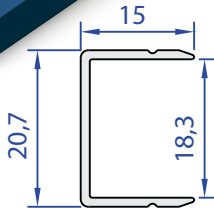
60210-00 0,151 Kg/m
