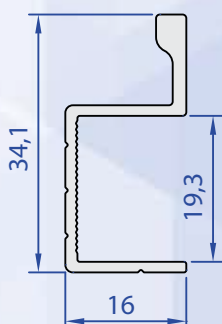
60389-00 0,284 Kg/m
