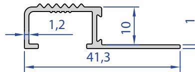
60085-00 0,223 kg/m
