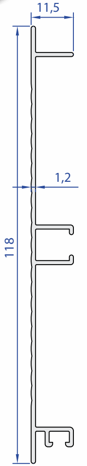
60357-00 0,527 Kg/m
