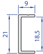
60364-00 0,138 Kg/m
