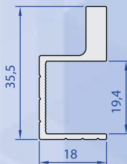
60377-00 0,430 Kg/m
