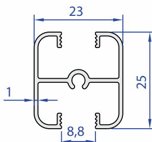
60440-00 0,292 Kg/m
