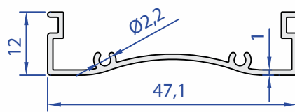
60132-00 0,238 kg/m
