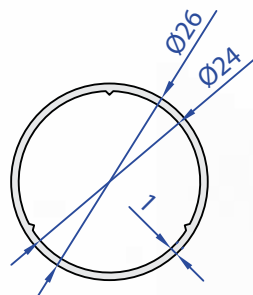
60014-00 0,215 kg/m
