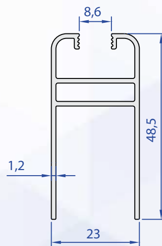
60177-00 0,496 kg/m
