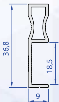
60365-00 0,269 Kg/m
