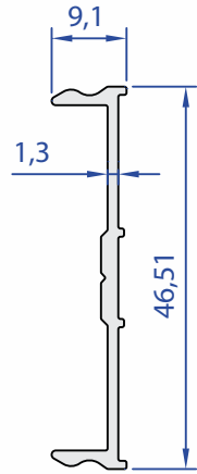
05716-00 0,251 Kg/m
