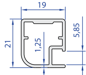
60180-00 0,293 kg/m
