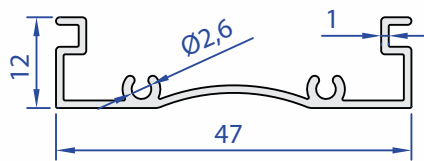
60041-00 0,266 kg/m
