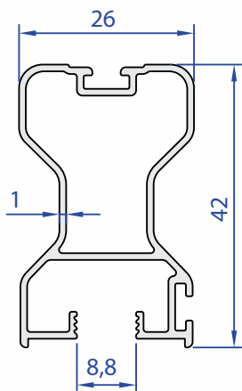
60442-00 0,455 Kg/m
