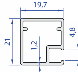
60276-00 0,286 Kg/m
