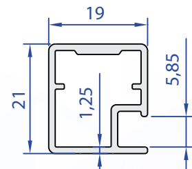
60211-00 0,300 Kg/m
