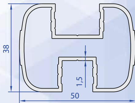
60043-00 0,910 kg/m
