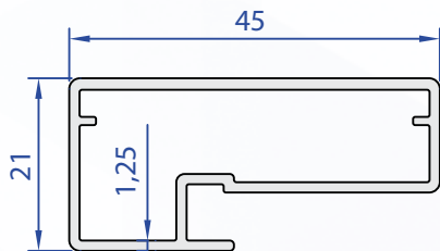
60224-00 0,480 Kg/m
