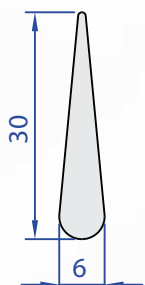
60015-00 0,292 kg/m
