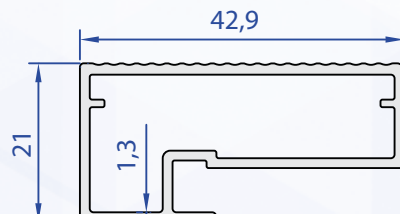
60450-00 0,477 Kg/m
