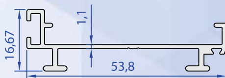
60149-00 0,337 Kg/m
