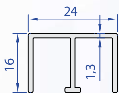
60136-00 0,250 kg/m
