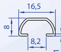
60110-00 0,086 kg/m
