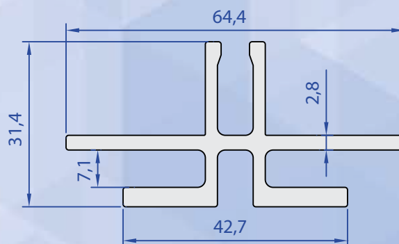
60126-00 1,181 kg/m
