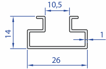
60451-00 0,192 Kg/m
