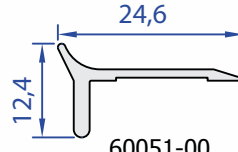
60051-00 0,129 kg/m
