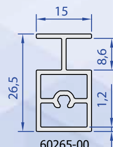
60265-00 0,328 Kg/m
