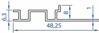
60073-00 0,209 kg/m
