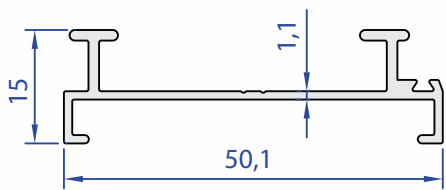
60425-00 0,308 Kg/m
