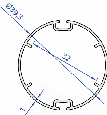
60437-00 0,405 Kg/m
