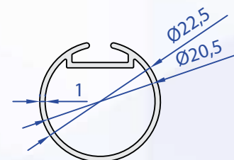
60040-00 0,212 kg/m
