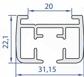
05074-00 0,545 kg/m
