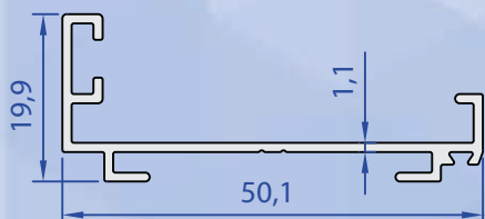
60146-00 0,306 Kg/m
