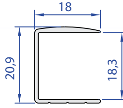
60430-00 0,159 Kg/m
