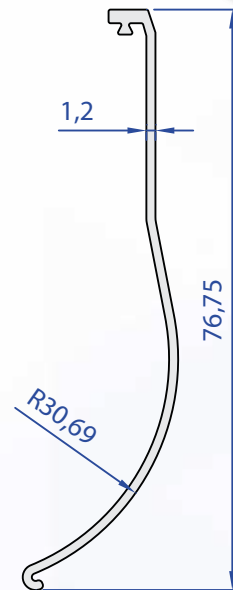
60402-00 0,307 Kg/m
