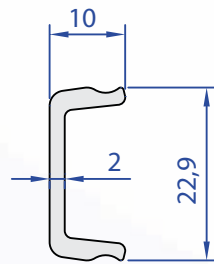
60571-00 0,210 Kg/m
