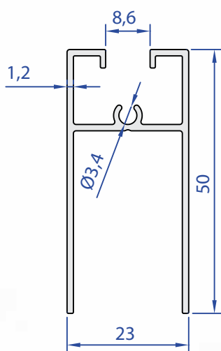
60175-00 0,466 kg/m
