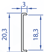
60445-00 0,064 Kg/m
