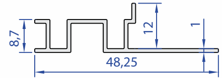
60075-00 0,239 kg/m
