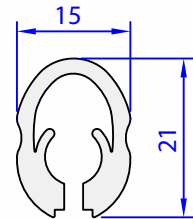
05022-00 0,373 kg/m
