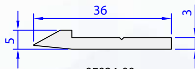
05024-00 0,296 kg/m
