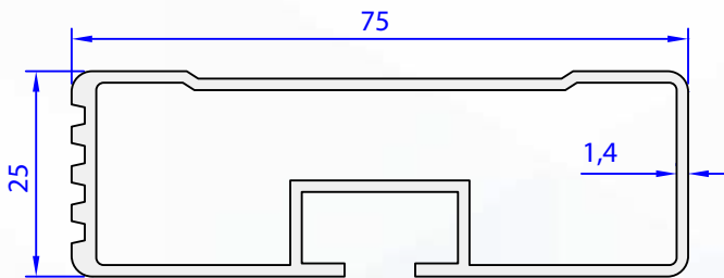
06499-00 0,905 Kg/m
