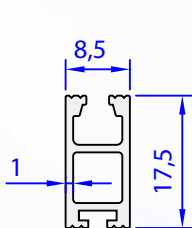
05420-00 0,179 kg/m
