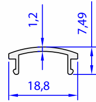
05062-00 0,095 kg/m
