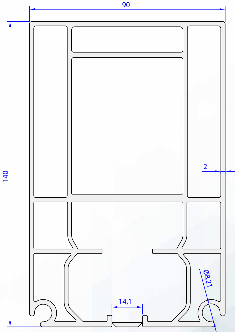
07014-00 5,491 Kg/m
