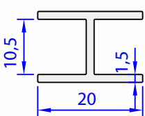
05118-00 0,205 kg/m
