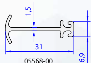
05568-00 0,218 kg/m
