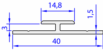
05617-00 0,233 kg/m
