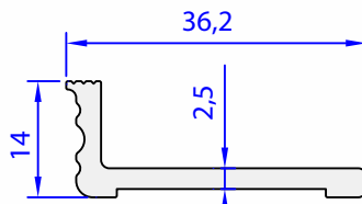
05416-00 0,339 kg/m
