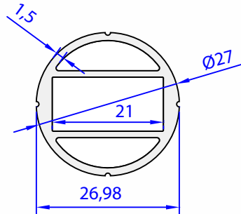
05130-00 0,523 kg/m
