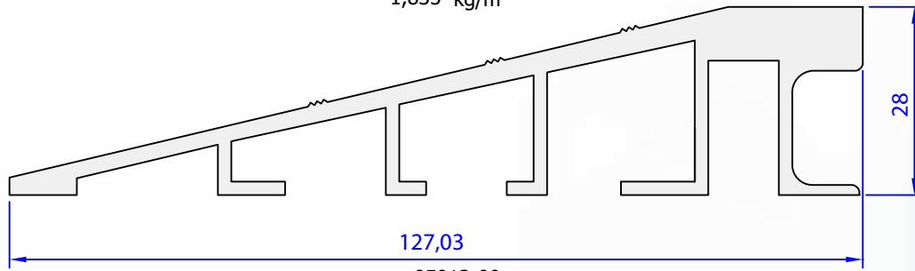
05013-00 2,045 kg/m
