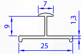
05430-00 0,147 kg/m
