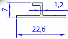
05378-00 0,104 kg/m
