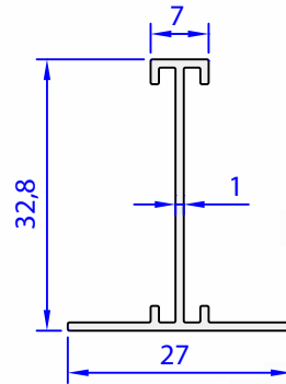
05210-00 0,197 kg/m
