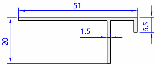
05504-00 0,303 kg/m
