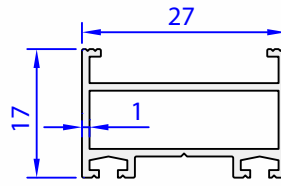
05157-00 0,269 kg/m
