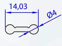
05079-00 0,101 kg/m
