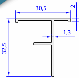
05640-00 0,258 kg/m
