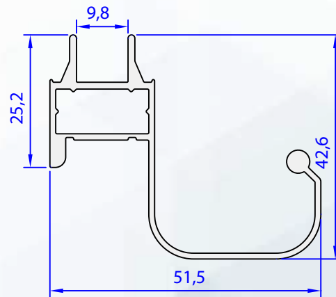
05241-00 0,540 kg/m
