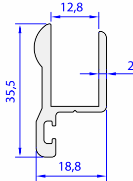
05205-00 0,477 kg/m
