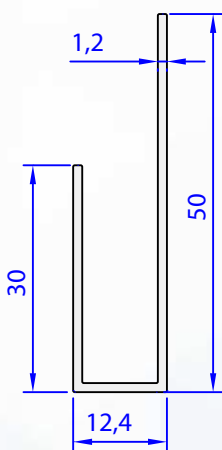
05153-00 0,293 kg/m
