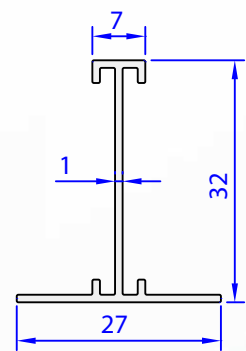
05161-00 0,195 kg/m
