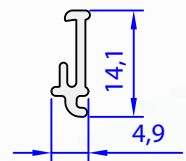
05569-00 0,076 kg/m
