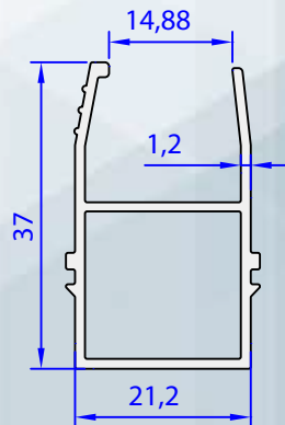
05344-00 0,381 kg/m
