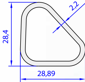
05043-00 0,515 kg/m
