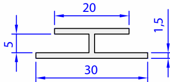
05083-00 0,224 kg/m
