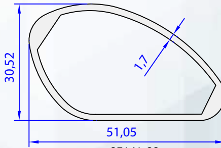
05141-00 0,672 kg/m
