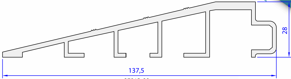
05012-00 1,835 kg/m
