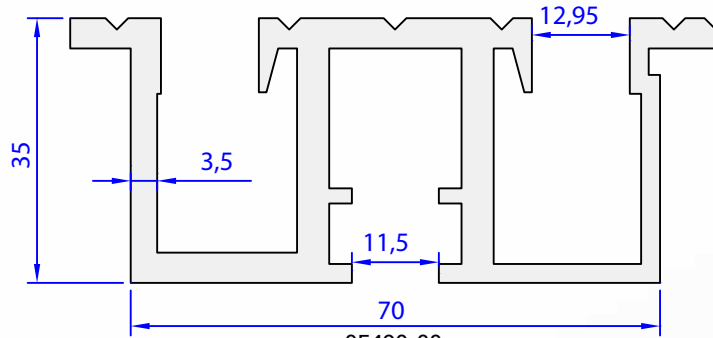
05490-00 2,313 kg/m
