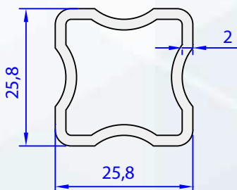
05016-00 0,515 kg/m
