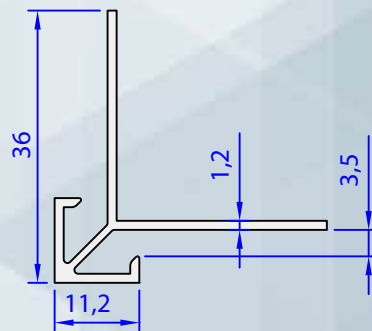
05376-00 0,291 kg/m
