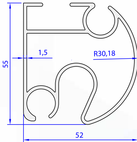
05021-00 1,162 kg/m
