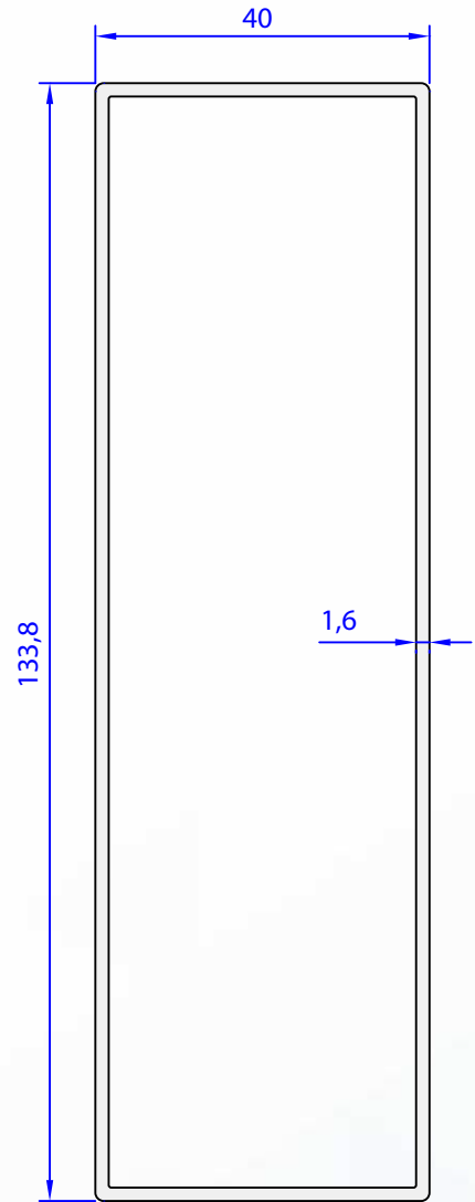
07016-00 1,477 Kg/m
