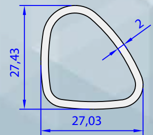
05266-00 0,446 kg/m
