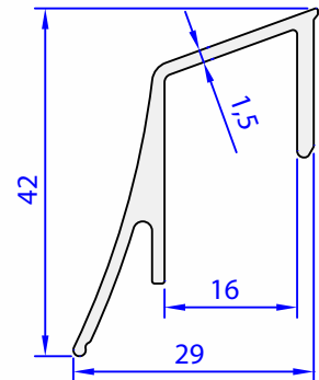
05421-00 0,411 kg/m
