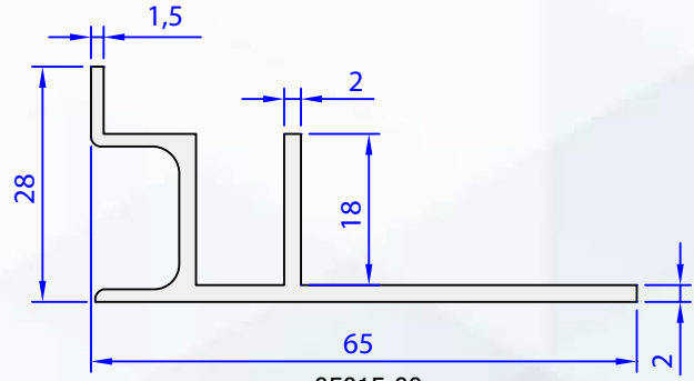
05015-00 0,616 kg/m
