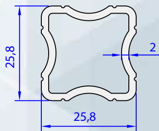
05050-00 0,506 kg/m
