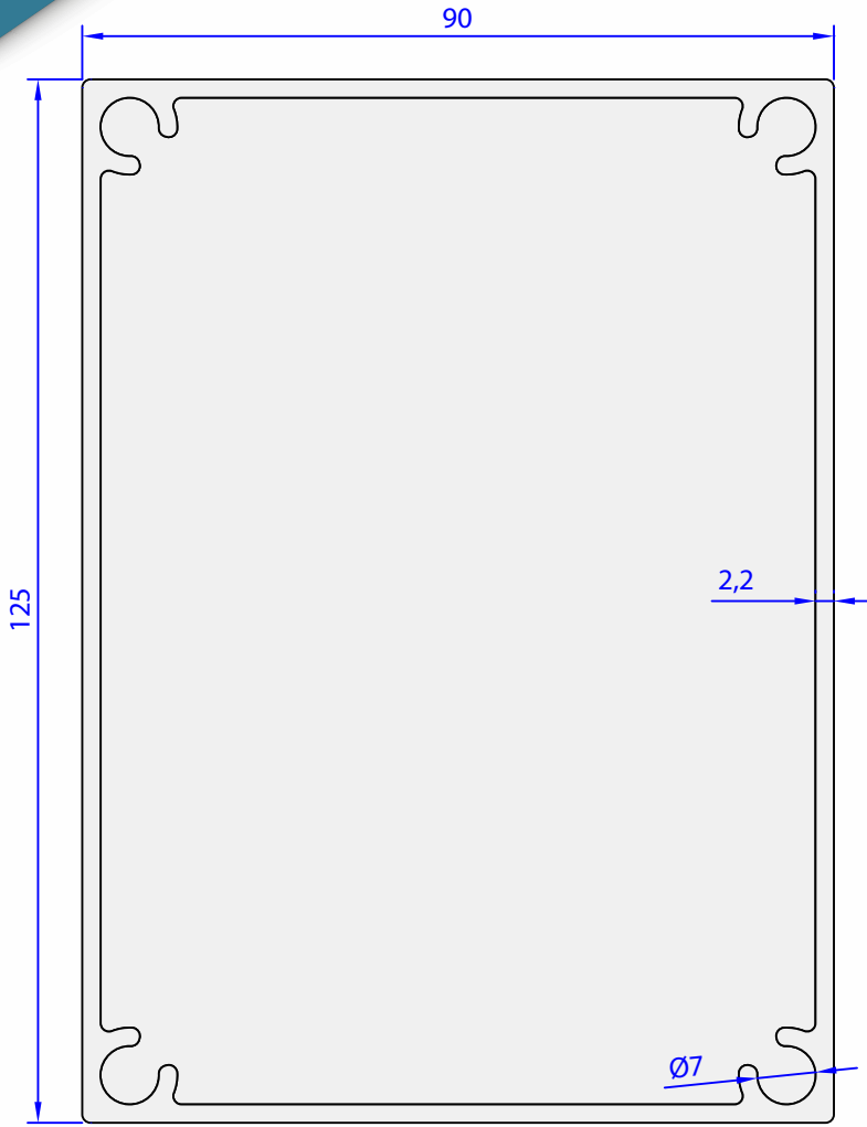
07015-00 2,791 Kg/m
