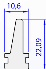
05017-00 0,357 kg/m
