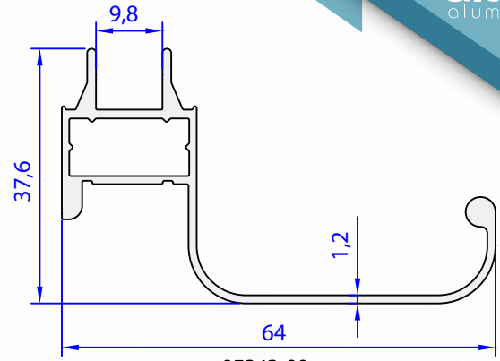
05343-00 0,564 kg/m
