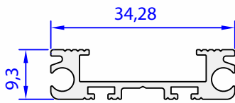
05078-00 0,290 kg/m
