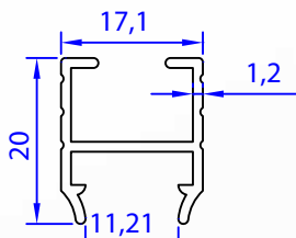
05073-00 0,205 kg/m
