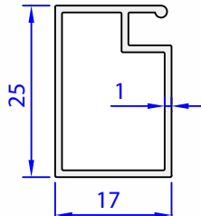
05109-00 0,234 kg/m
