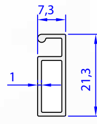
06770-00 0,150 Kg/m
