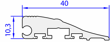
05113-00 0,503 kg/m
