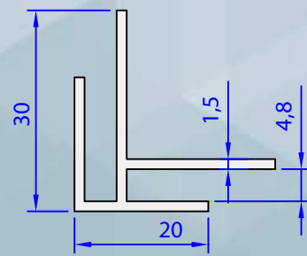
05058-00 0,363 kg/m
