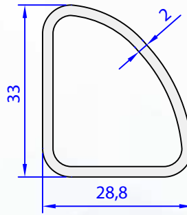
05128-00 0,533 kg/m
