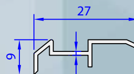
05068-00 0,109 kg/m
