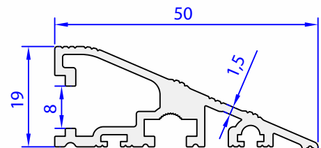
05429-00 0,602 kg/m
