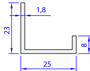
06487-00 0,256 Kg/m
