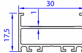
05462-00 0,288 kg/m
