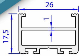
05002-00 0,309 kg/m
