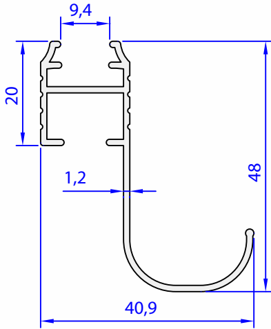
05148-00 0,395 kg/m
