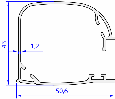
05108-00 0,594 kg/m
