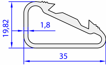
05008-00 0,516 kg/m
