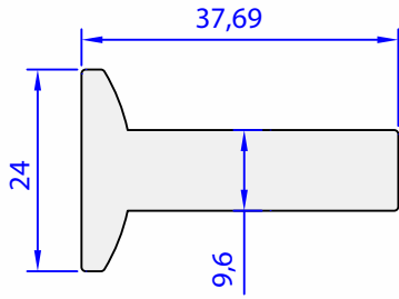
05060-00 1,147 kg/m
