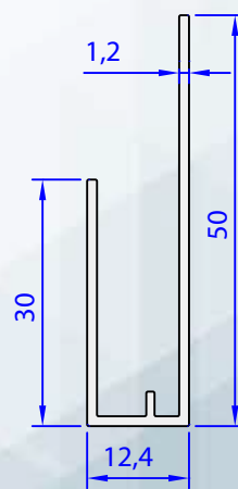
05189-00 0,301 kg/m
