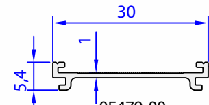
05479-00 0,113 kg/m
