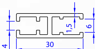
05082-00 0,336 kg/m
