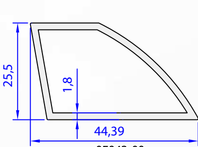
05042-00 0,555 kg/m
