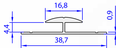
05235-00 0,188 kg/m
