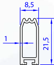
05037-00 0,166 kg/m
