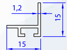
05025-00 0,118 kg/m
