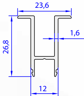
05358-00 0,283 kg/m
