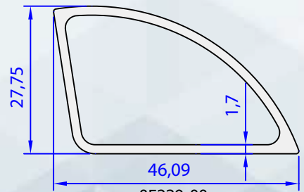
05239-00 0,564 kg/m
