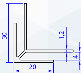
05353-00 0,304 kg/m
