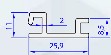
05185-00 0,290 kg/m
