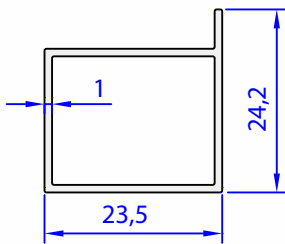
05471-00 0,234 kg/m
