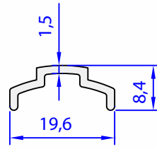
05061-00 0,121 kg/m
