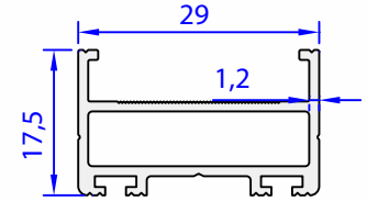
05329-00 0,324 kg/m
