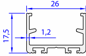
05054-00 0,265 kg/m
