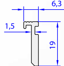
05418-00 0,154 kg/m
