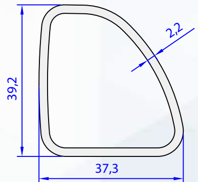
05360-00 0,733 kg/m
