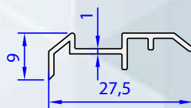
05621-00 0,120 kg/m
