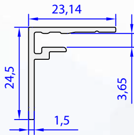
05514-00 0,224 kg/m
