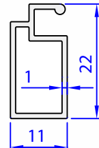
05110-00 0,179 kg/m
