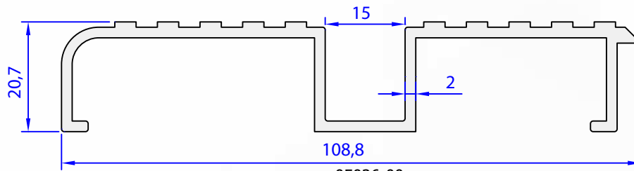
05026-00 1,099 kg/m
