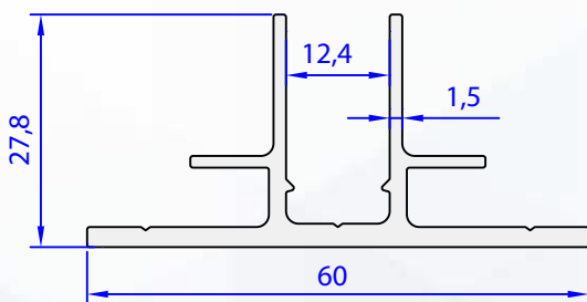
05359-00 0,717 kg/m
