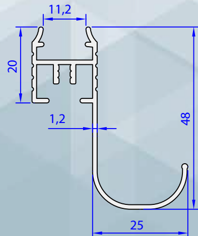
05064-00 0,423 kg/m
