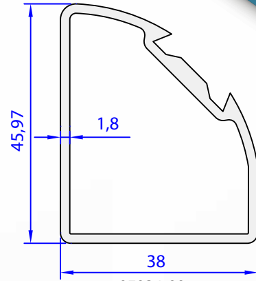
05034-00 0,782 kg/m
