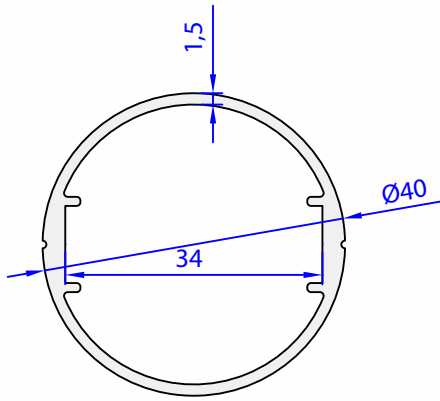
05063-00 0,593 kg/m
