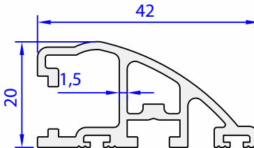
05003-00 0,575 kg/m
