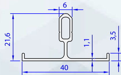
05546-00 0,260 kg/m
