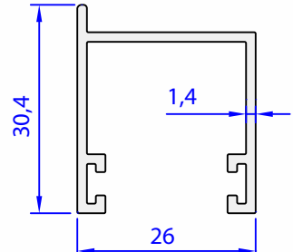
05169-00 0,362 kg/m
