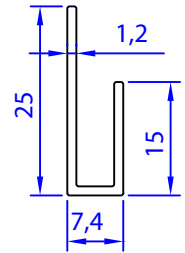
06497-00 0,146 Kg/m
