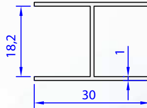
05577-00 0,212 kg/m
