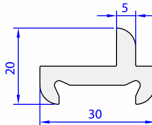
05548-00 0,608 kg/m
