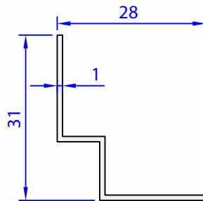
05409-00 0,157 kg/m
