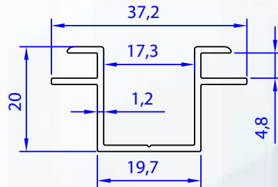
05580-00 0,278 kg/m
