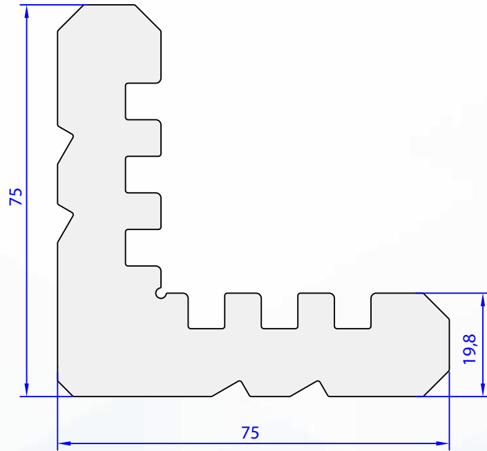
05424-00 5,928 kg/m
