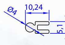
05114-00 0,090 kg/m
