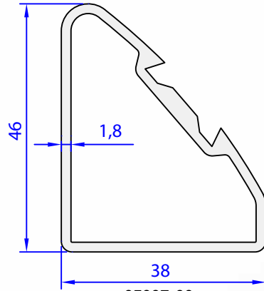
05007-00 0,768 kg/m
