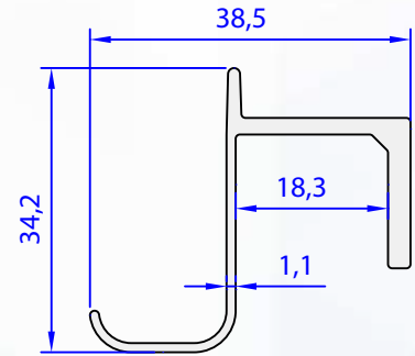
05565-00 0,394 kg/m
