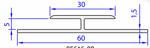
05616-00 0,382 kg/m
