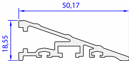
05188-00 0,557 kg/m
