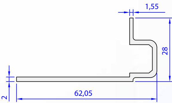
05014-00 0,513 kg/m
