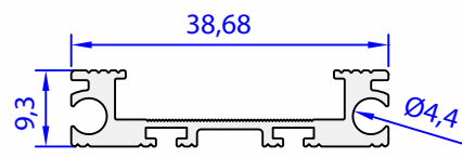
05560-00 0,322 kg/m
