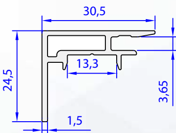
05512-00 0,331 kg/m
