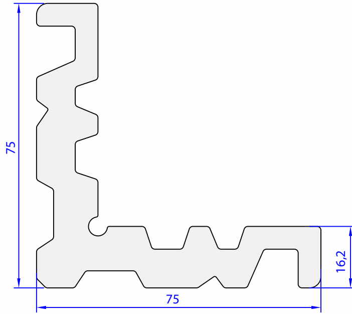
05582-00 4,186 kg/m
