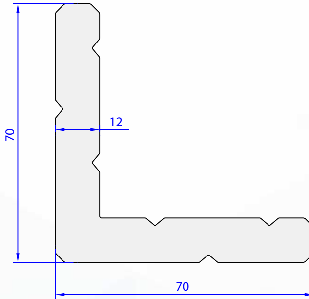
05622-00 4,034 kg/m
