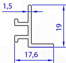
05420-00 0,179 kg/m
