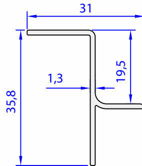
05508-00 0,230 kg/m
