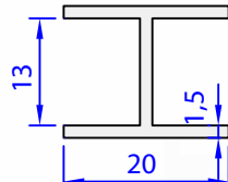
05304-00 0,215 kg/m
