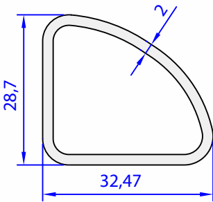
05167-00 0,528 kg/m
