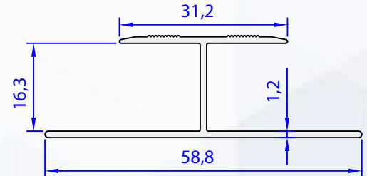
05653-00 0,346 kg/m
