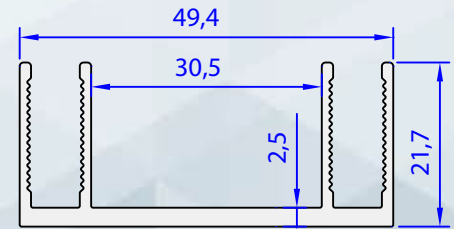
05264-00 0,593 kg/m
