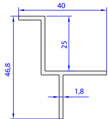
05581-00 0,414 kg/m
