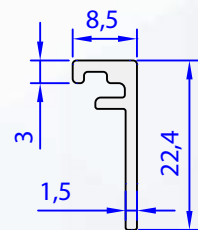
05513-00 0,152 kg/m
