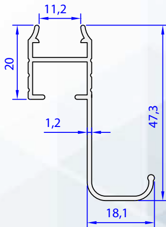
05072-00 0,356 kg/m
