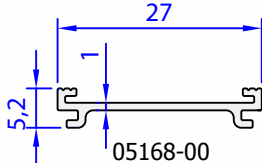
05168-00 0,111 kg/m
