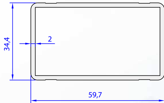
05020-00 0,945 kg/m
