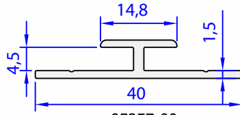
05257-00 0,241 kg/m
