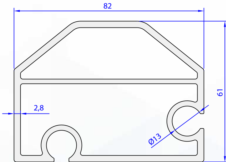
07013-00 2,613 Kg/m
